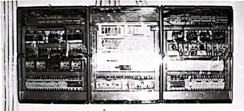
CUADRO DE MANIOBRA EQUIPOS FRIGORIFICOS (HOTEL TOPACIO - MENORCA)
