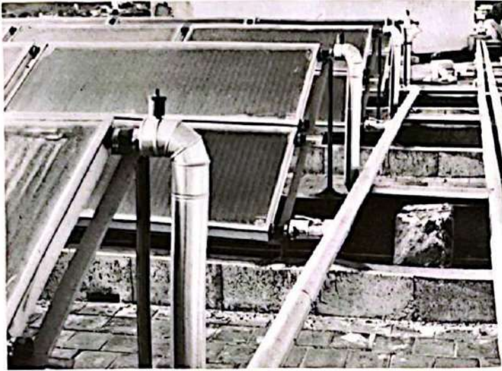
INSTALACION DE ENERGIA SOLAR PARA A.C.S. (HOTEL AGAMENON - MENORCA)
