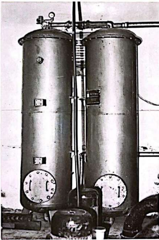
RECUPERACION DE AGUAS RESIDUALES ARENAL D'EN CASTELL - MENORCA
