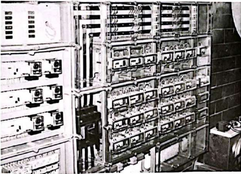
CUADROS DE MANIOBRA (COMPLEJO COMERCIAL - BINIBECA - MENORCA)
